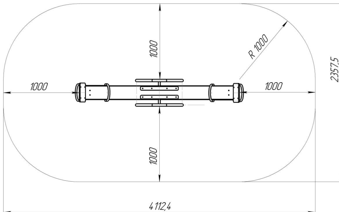
Рисунок 1- схема безопасности
